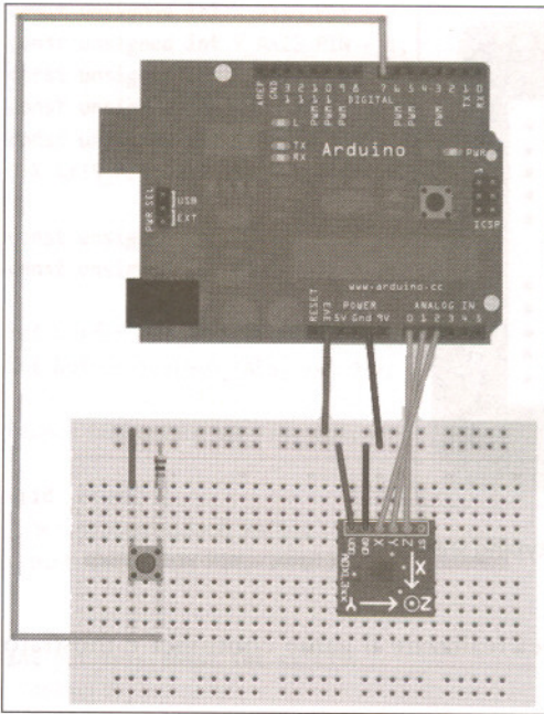
Figura 6.4 Game controller con accelerometro e pulsante.
