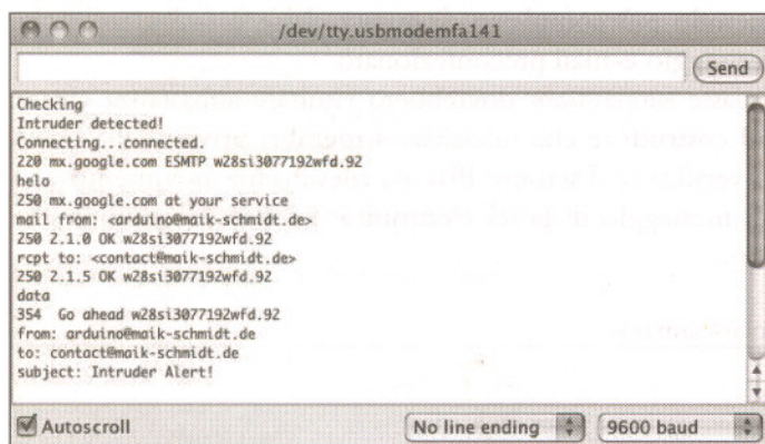
Figura 8.11 Output del sistema anti-intrusione.
