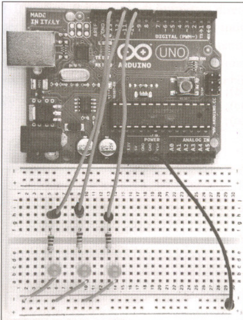
Figura 3.7 Prima versione funzionante del dado binario.
