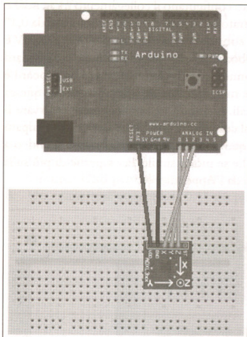
Figura 6.3 . Collegamenti tra sensore ADXL335 e scheda Arduino.
