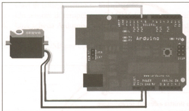
Figura 10.3 Schema di cablaggio per il collegamento di un servomotore a 5V.
