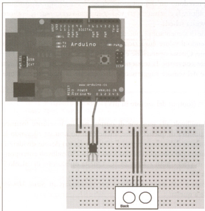
Figura 5.7 I sensori TMP36 e PING)) lavorano all'unisono.
