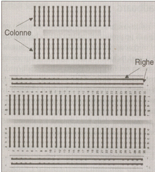
Figura 3.3 Collegamenti interni alla breadboard.
