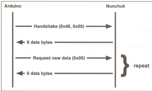
Figura 7.4 Flusso dei messaggi tra Arduino e Nunchuk.
