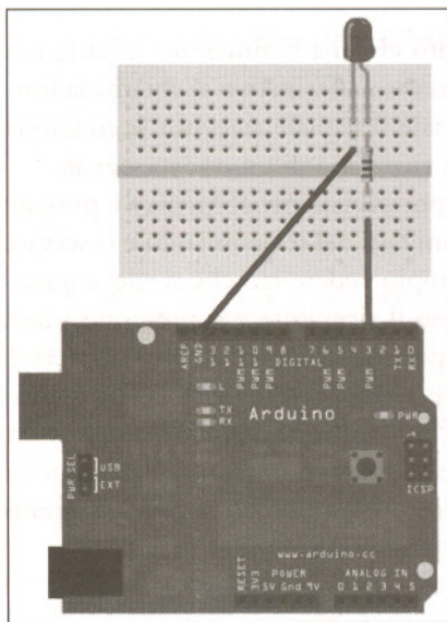
Figura 9.6 Collegamento tra Arduino e led a infrarossi.
