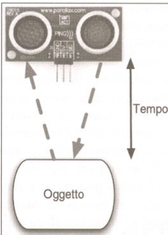
Figura 5.2 Principio di funzionamento del sensore PING))).
