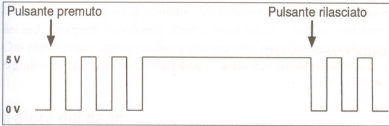
Figura 3.9 Rimbalzi del segnale elettrico prodotti da un pulsante.
