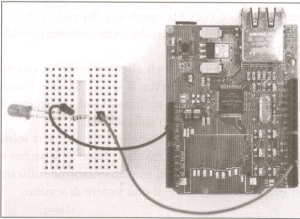
Figura 9.8 Telecomando controllato via Ethernet.
