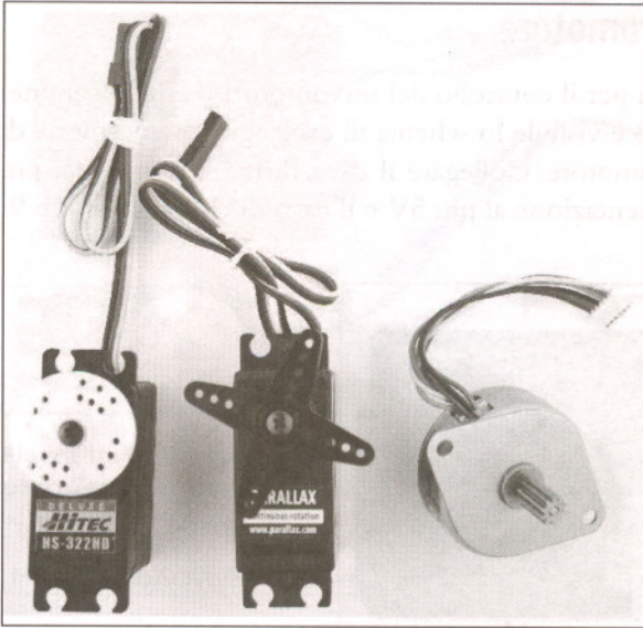
Figura 10.2 Tipi di motore (da sinistra a destra): servomotore standard, motore a rotazione continua, motore passo-passo.
