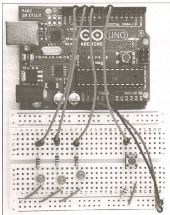
Figura 3.10 Il dado binario con pulsante esterno.
