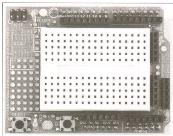
Figura 6.5 Esempio di scheda Arduino Prototyping shield.
