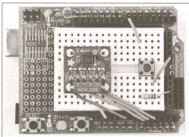
Figura 6.6 Prototipo completo del game controller su una scheda Proto shield.
