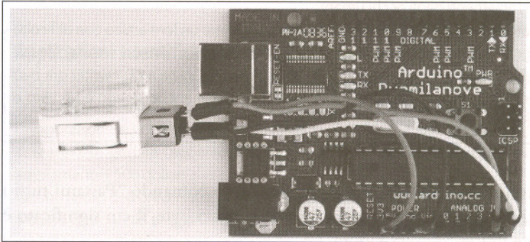
Figura 7.2 Collegamento tra Nunchuk e scheda Arduino.
