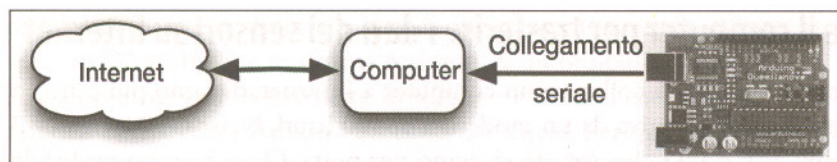
Figura 8.2 Collegamento tra Arduino e Internet tramite computer.
