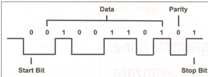
Figura C.1 Comunicazione seriale a livello di bit.
