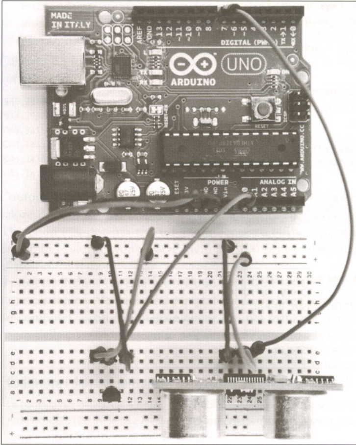
Figura 5.8 Foto del circuito definitivo.
