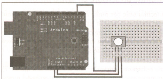
Figura 8.8 Schema di principio del circuito di cablaggio di un sensore PIR.
