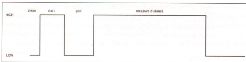
Figura 5.4 Diagramma temporale del segnale del sensore PING)).
