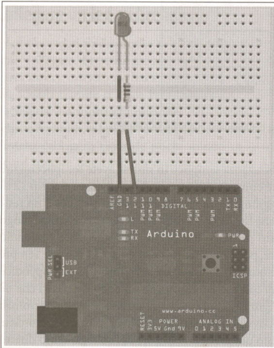
Figura 3.6 Potete utilizzare l'intera estensione di una breadboard.
