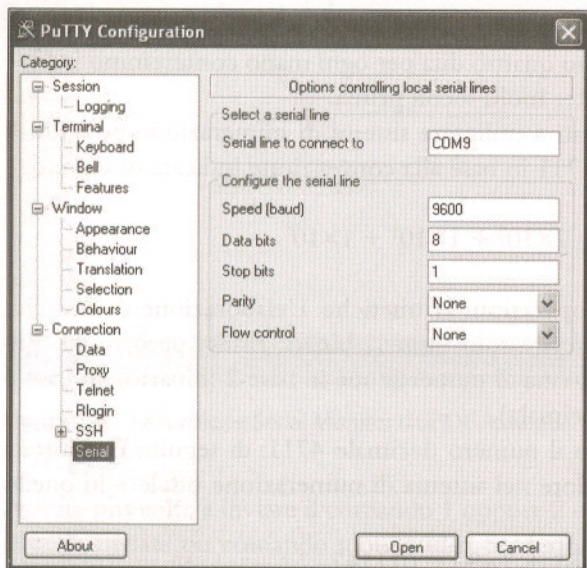
Figura 2.5 Configurazione di Putty per utilizzare questo sistema di monitoraggio con Arduino.
